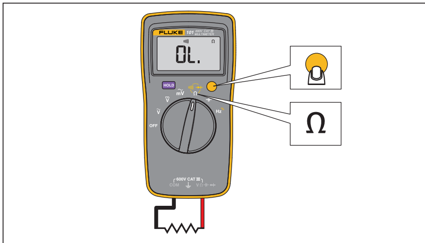
圖 3. 測量電阻/連續性
