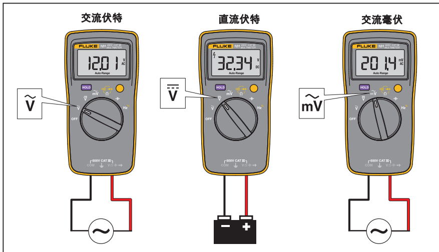
圖 2. 測量交流和直流電壓
