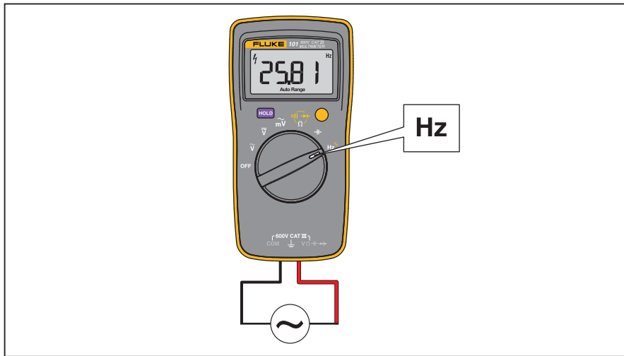
圖 4. 測量頻率/工作週率
