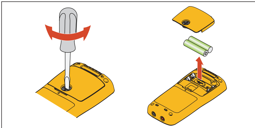
圖 5。更換電池
