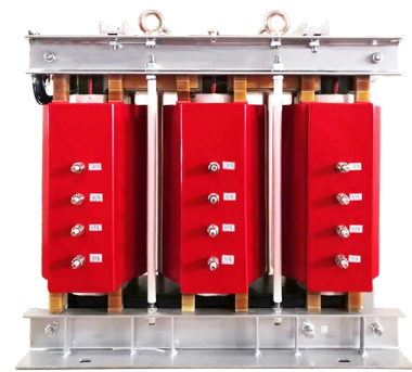
馬達啟動補償器
