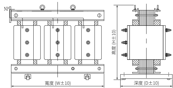
馬達啟動補償器
