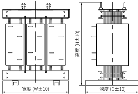
馬達啟動電抗器
