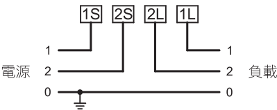
BAW-2A 單相三線式
