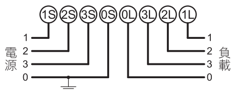
用於三相四線式電源
