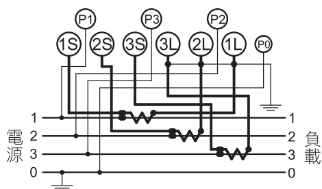
用於三相四線式電源
