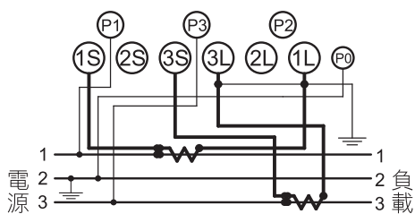
用於三相三線式電源
