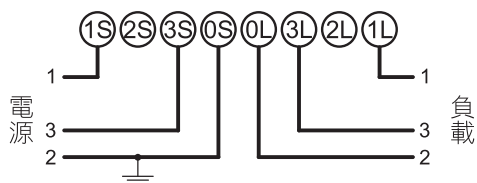
用於三相三線式電源
