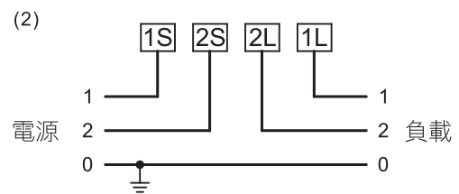
BAW-2D 單相三線式
