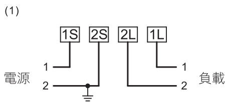
BAW-1D 單相二線式
