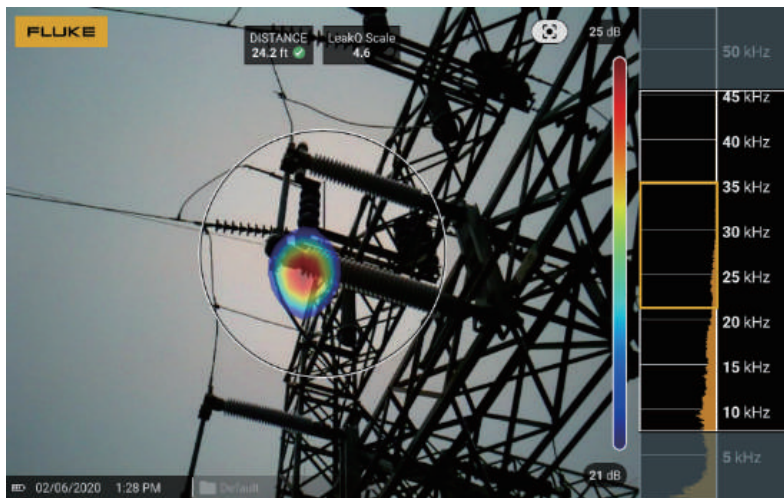
避雷器，斷路器，絕緣礙子 - 絕緣狀態監測
